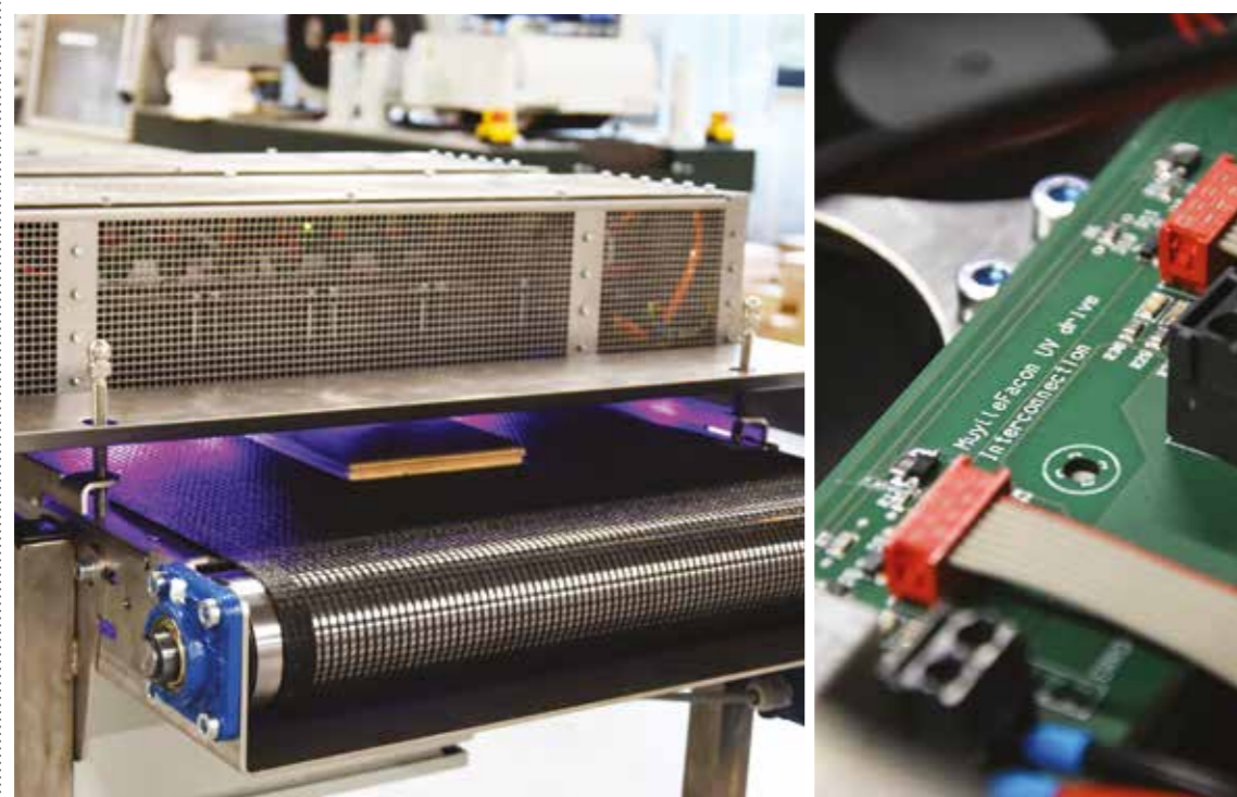
(Foto: LED-curing industry unit, instalada en el Rubio® Monocoater.)
